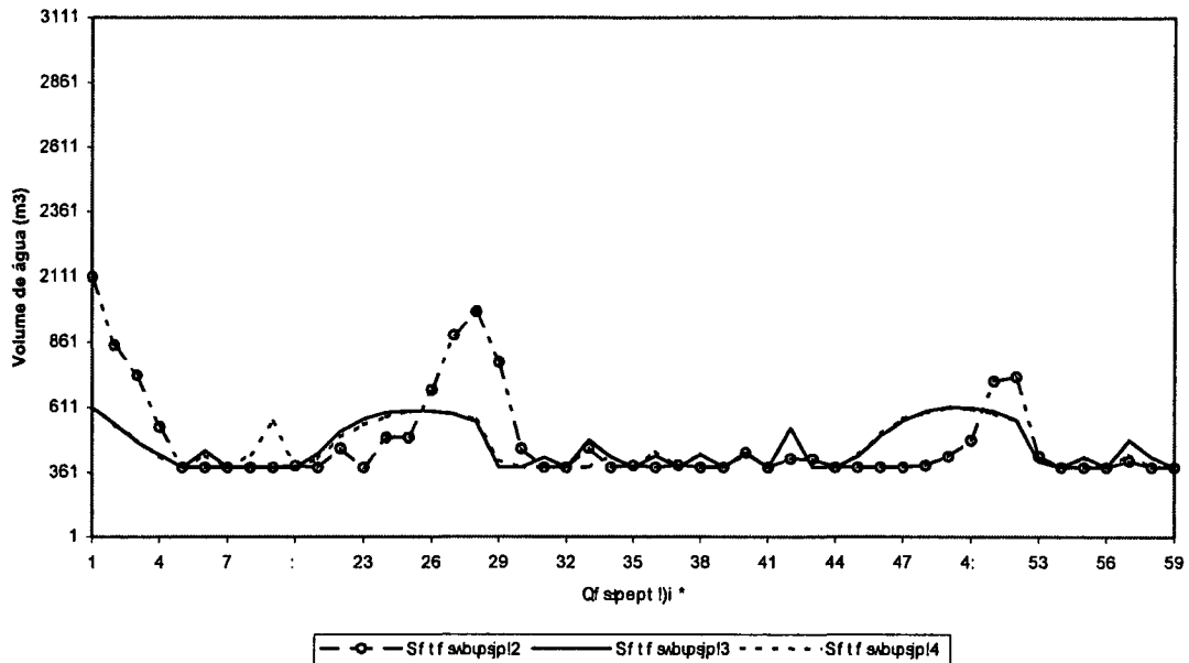
Figura 12 – Volume dos reservatórios com T = 2 (Modelo Inteiro).
