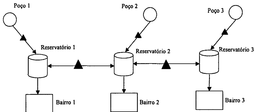
Figura 1. Exemplo de uma rede de abastecimento.
