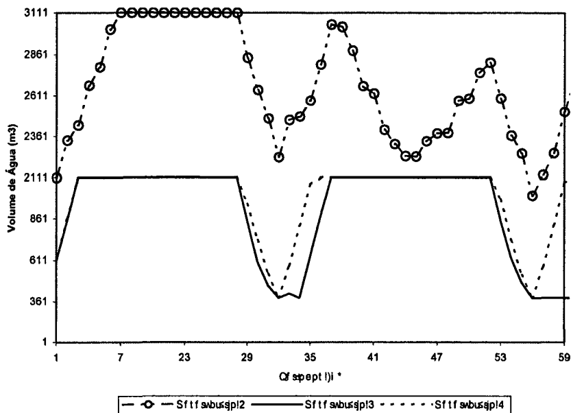
Figura 7 – Volume dos reservatórios nos dois primeiros dias para T = 7 (Modelo Linear).
