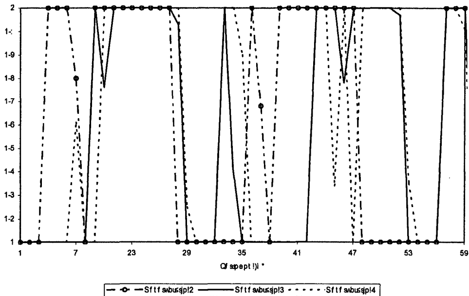
Figura 10 – Política de operação das bombas (Modelo Inteiro).
