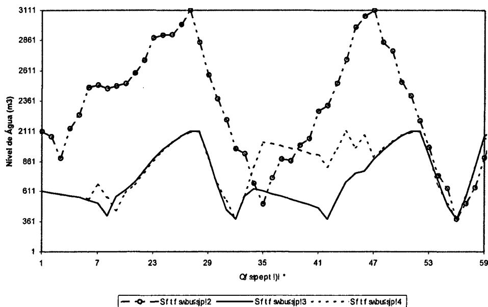
Figura 9 – Volume dos reservatórios para dois dias com T = 7 (Modelo Inteiro).
