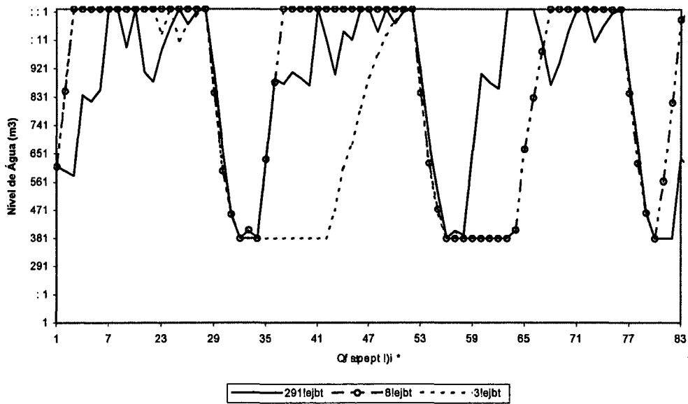
Figura 5. Volume de água no reservatório 2.
