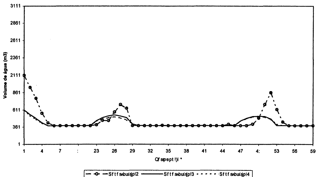
Figura 11 – Volume dos reservatórios com T = 2 (Modelo Linear).
