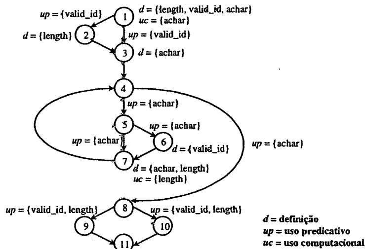
Figura 3. Grafo Def-Use do programa identifier .
