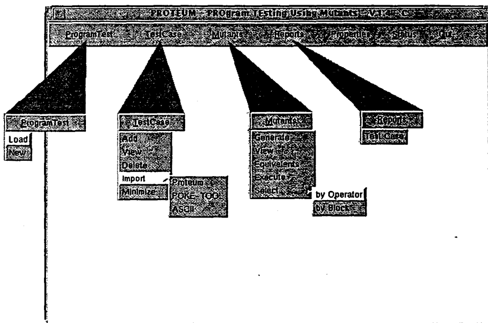
Figura 7. Operações disponíveis na interface da Proteum .
