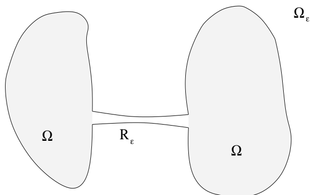
FIG. 1. Dumbbell domain
